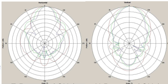
E-Plane (1-2GHz)
