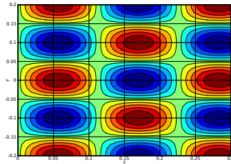
(b) 2 GHz
