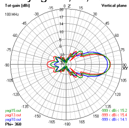
yagi 10,13,15
